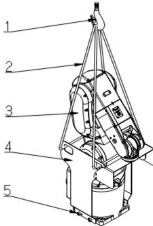
①：天車 ②：吊繩 ③ 吊裝限位支架 ④ 吊裝支架 ⑤ 固定螺絲
